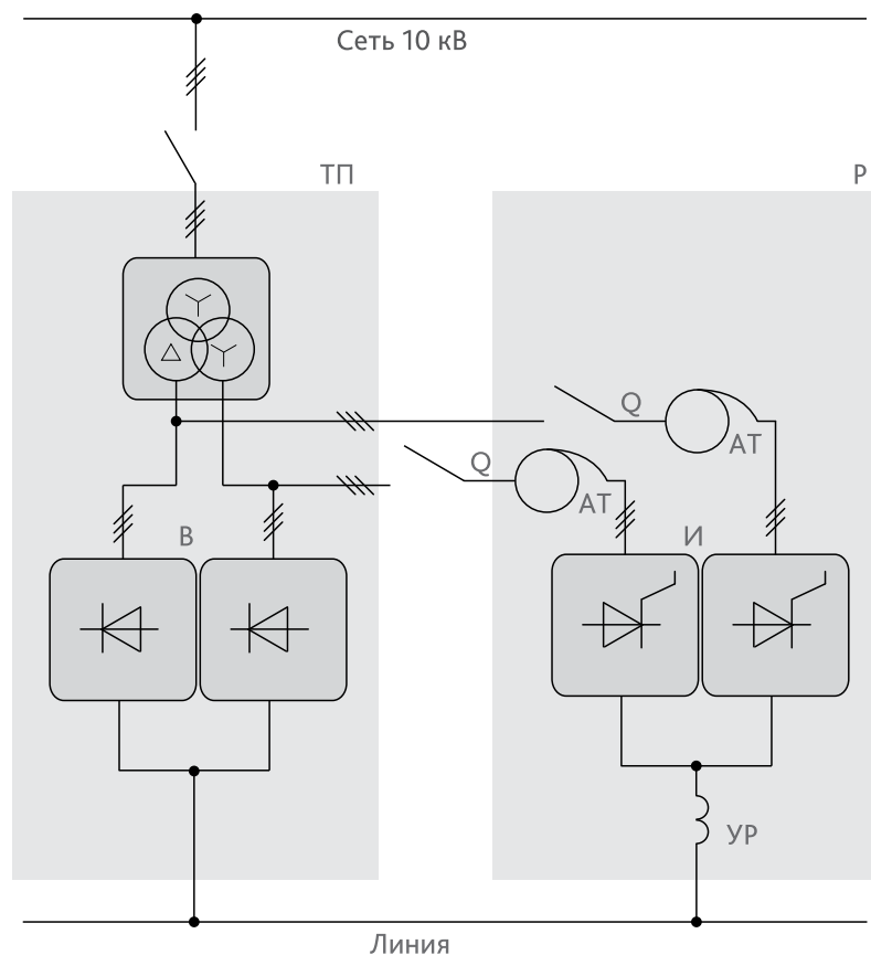
▲ Автотрансформаторная схема подключения рекуператора
