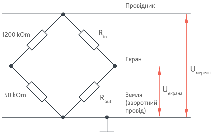
▲ Вимірвальна схема
