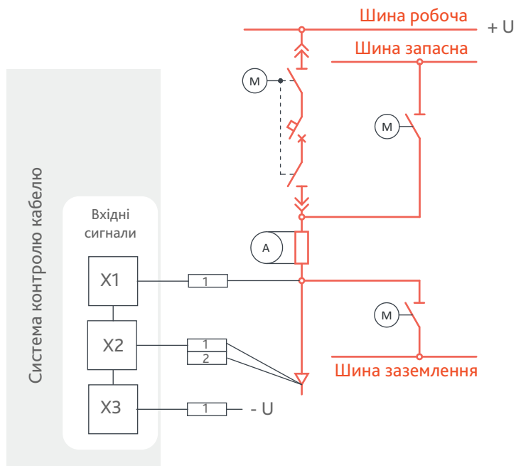
▲ Схема підключення системи контролю кабелю до розподільчого пристрою
