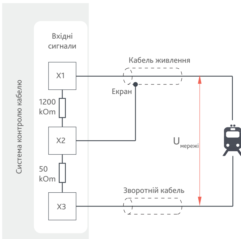
▲ Схема підключення до модуля системи контролю кабелю
