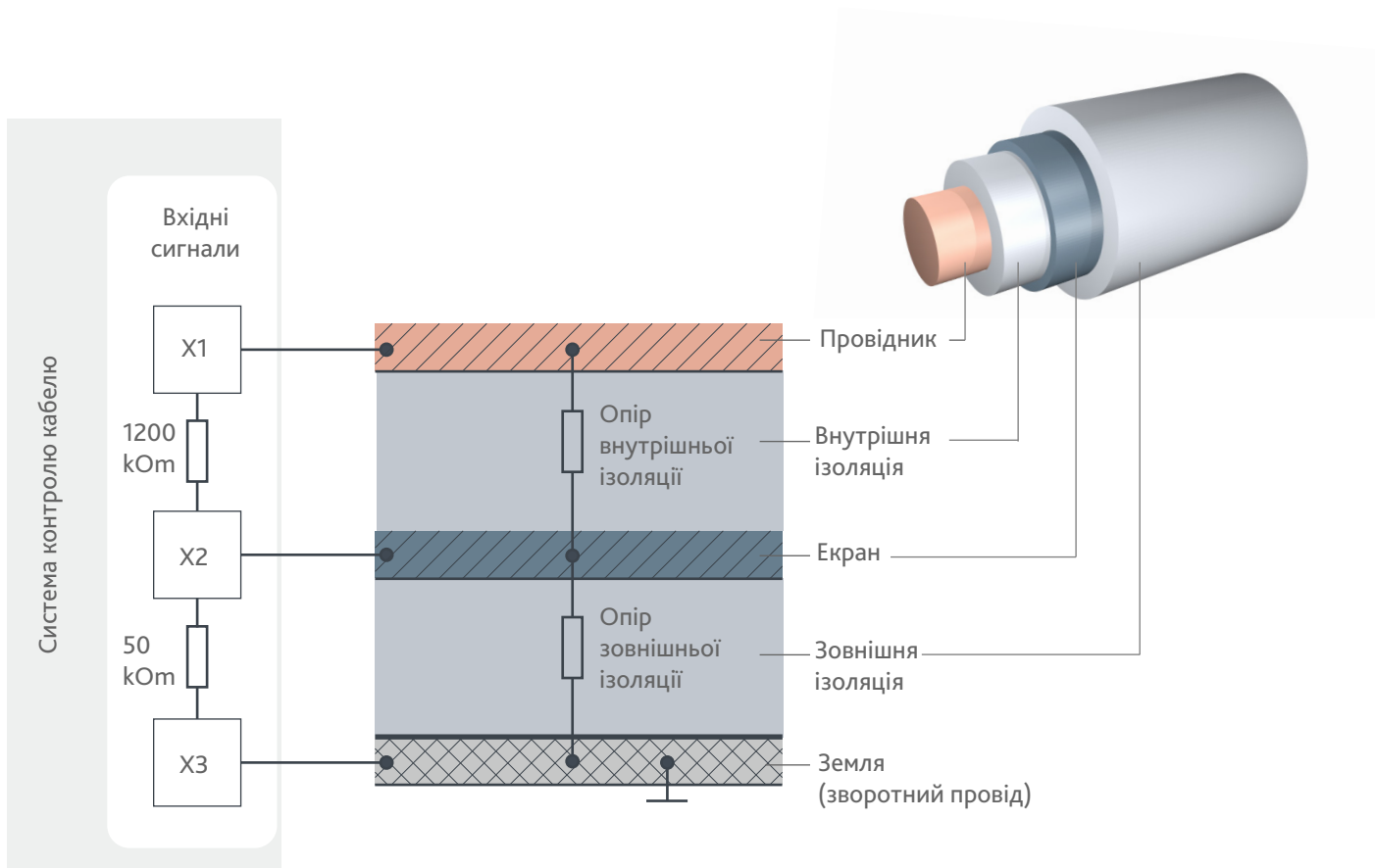
▲ Схема підключення кабелю до модуля системи контролю кабелю
