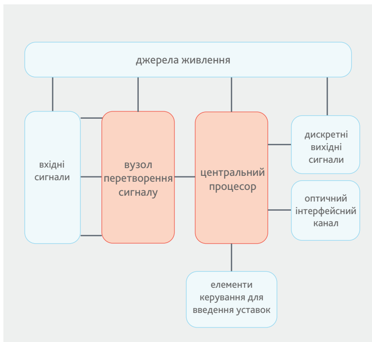
▲ Структурна схема системи контролю кабелю
